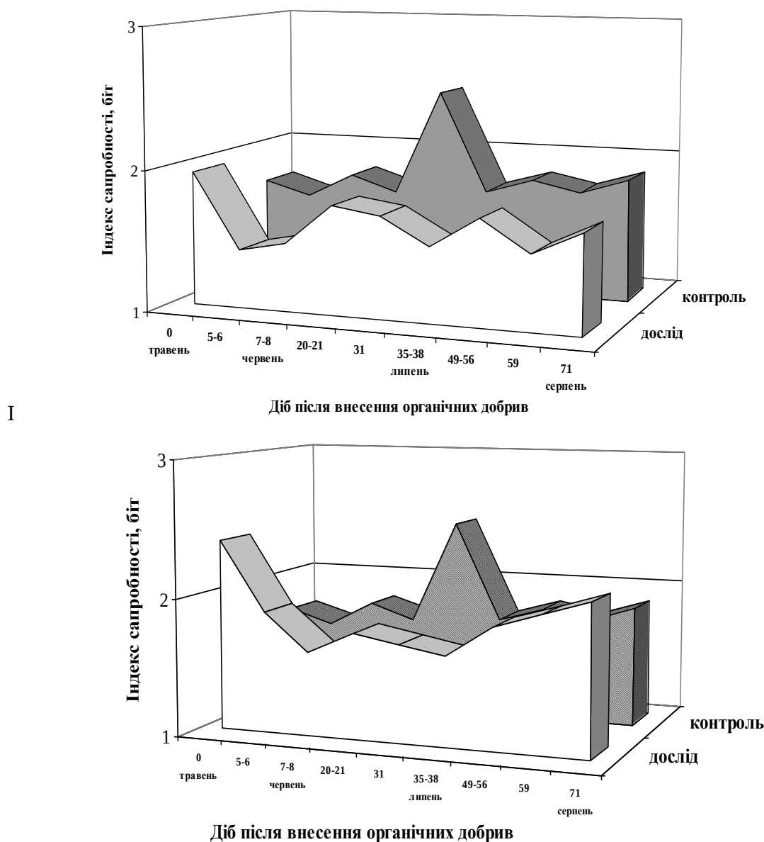
Рис. 2. Динаміка індексу сапробності за зоопланктоном у вирощувальних ставах: I, II, III – дослідні варіанти удобрення ставів у порівнянні з контролем.
