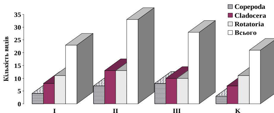
Рис. 1. Кількість індикаторних видів основних груп зоопланктону представлених у вирощувальних ставах удобрених зерновою бардою: I, II, III – дослідні варіанти удобрення ставів у порівнянні з контролем (К).
