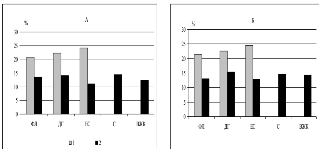
Рис. 2. Уміст основних фракцій поверхневих ліпідів в асиміляційних органах деревних рослин зони сильного забруднення ЗАТ «Криворізький суриканий завод» у фазу повного відособлення листка (А) та на 5-10 добу фази завершення росту листка (Б) в % від загальної суми: 1 – Populus italica , 2 – Betula pendula , ФЛ – фосфоліпіди, ДГ – дигліцериди, ЕС – етери стеринів, С – стерини, ВЖК – вільні жирні кислоти.
